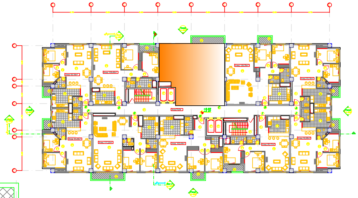
پلان مبلمان طبقه ۱-۸
